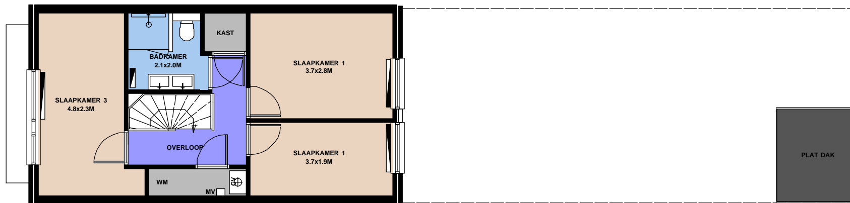
1E VERDIEPING
