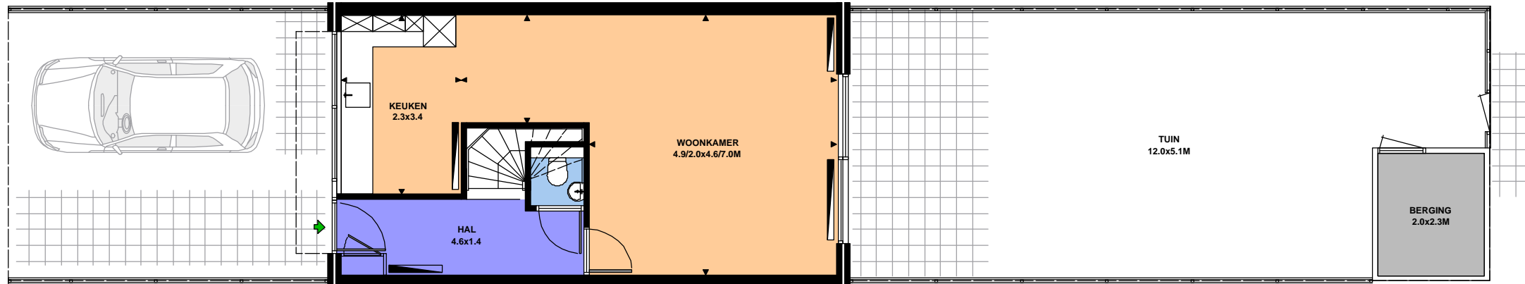
BEGANE GROND
