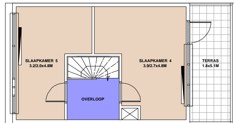
2E VERDIEPING
